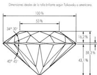
talla brillante proporciones
